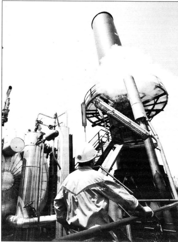
Nueva planta de hidrógeno para combustible de Enel Spa, dentro de la planta Andrea Palladio en Venecia, Italia. La capacidad de producción permitirá generar 60 millones de kilovatios/hora, suficientes para cubrir la demanda de 20 mil hogares, evitando la emisión de dióxido de carbono ■ Foto Reuters
